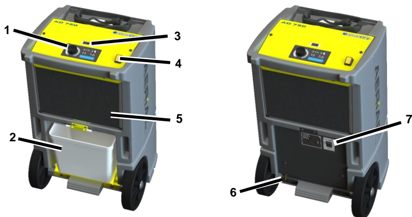
Fig. 2: Sett bakfra
