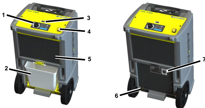
Fig. 2: Bakifrån
