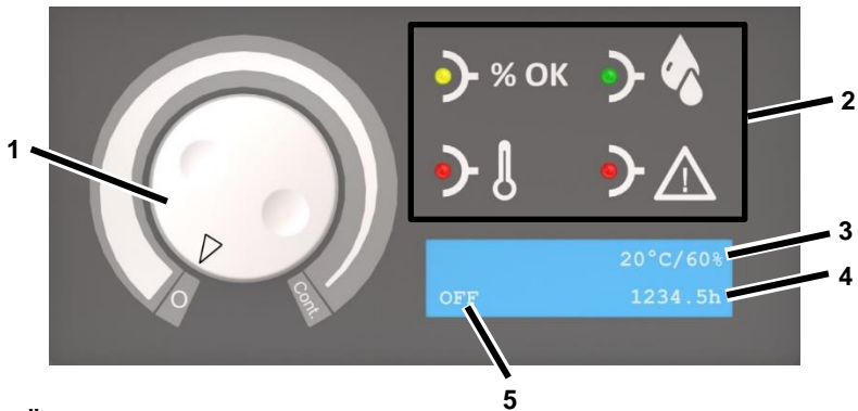
Fig. 3: Übersicht Bedienfeld
