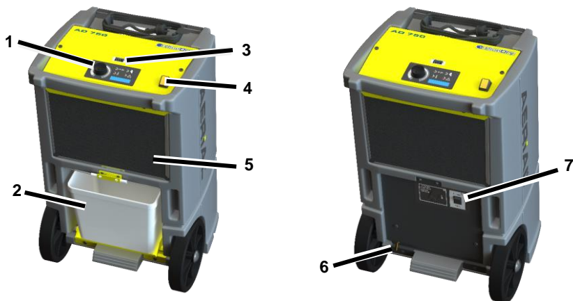
Afb. 2: Achteraanzicht
