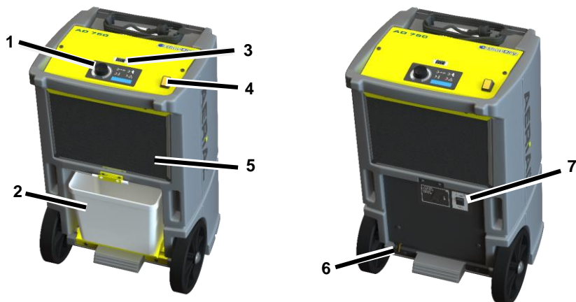
Rys. 2: Widok z tyłu
