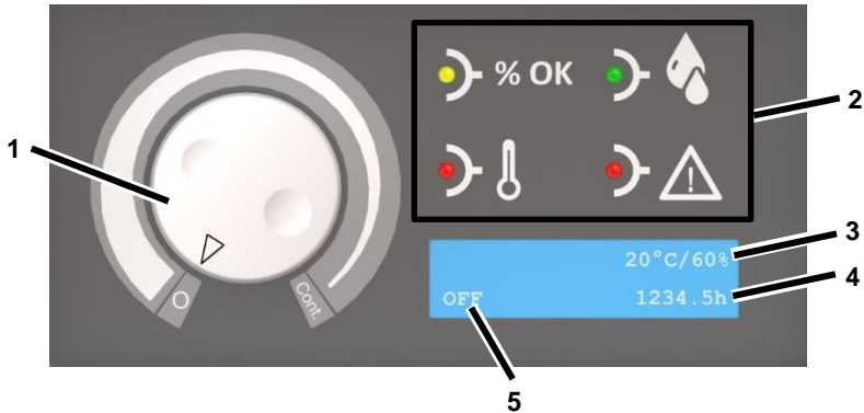
Afb. 3: Overzicht bedieningspaneel
