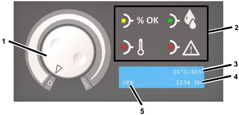
Kuva 3: Käyttöpaneelin yleiskuvaus
